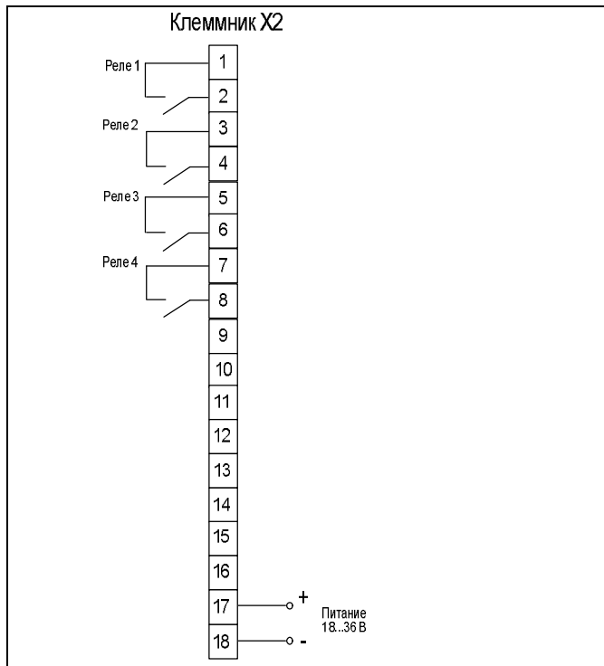
Рисунок 4е – Модификация MDS AIO-4/4R
