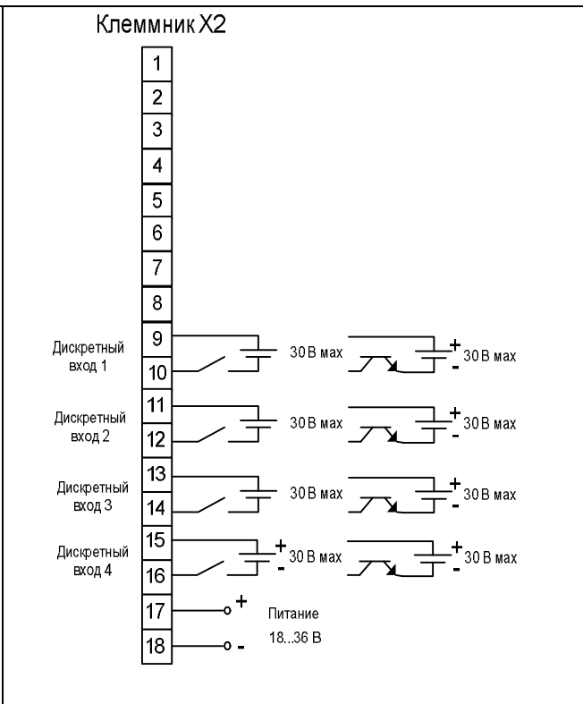
Рисунок 4б – Модификация MDS AIO-4/X
