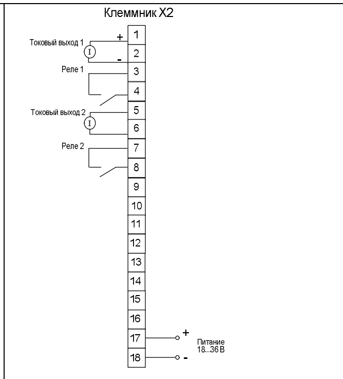
Рисунок 4ж – Модификация MDS AIO-4/2R
