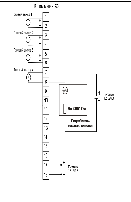
Рисунок 4г – Модификация MDS AIO-4/0R-
