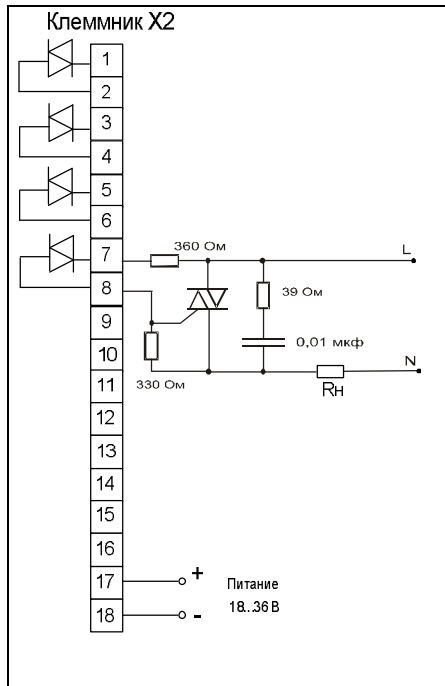
Рисунок 4в – Модификация MDS AIO-4/4S
