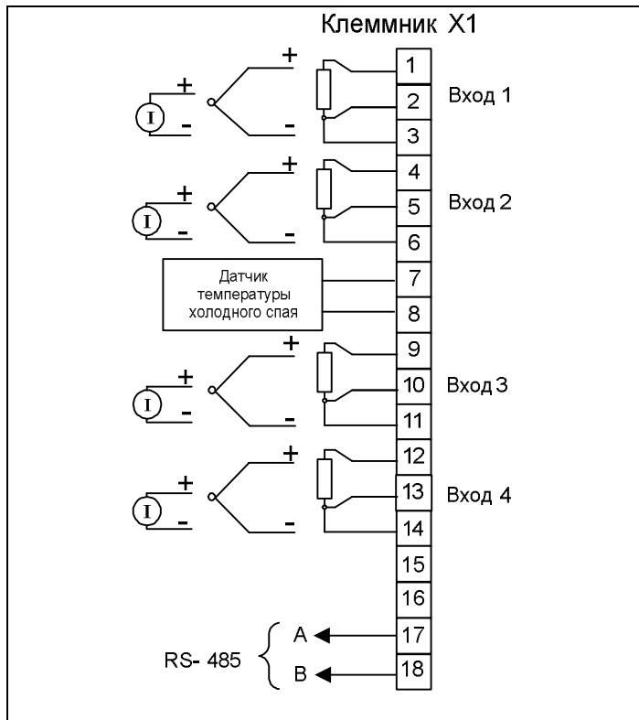
Рисунок 4а – Модификация MDS AIO-4/X
