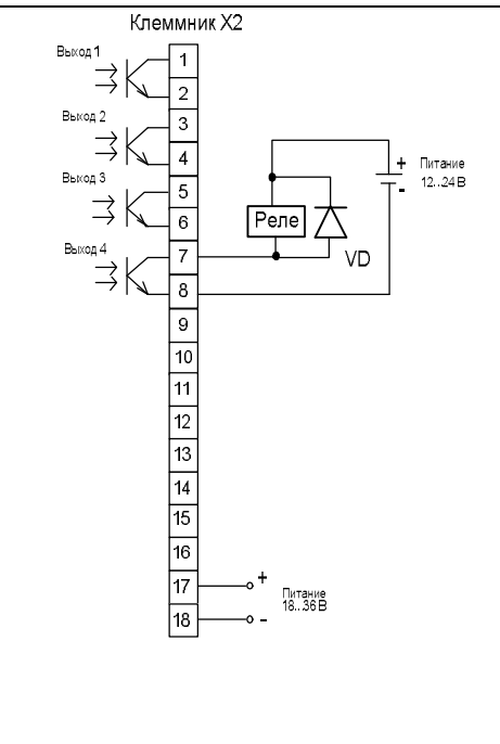
Рисунок 4д – Модификация MDS AIO-4/4T
